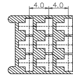
A-A SEC
