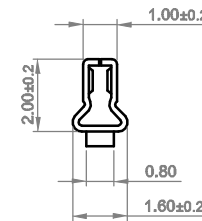
Sec:B-B
