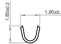
Sec:A-A
