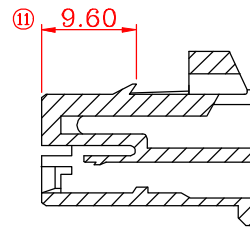
SEC A-A
