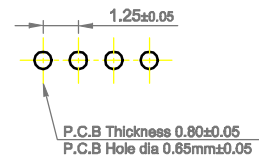
P.C.B. LAYOUT
